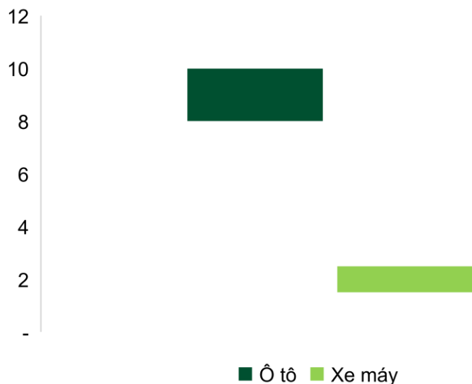
Mức tiêu hao nhiên liệu (lít/100 km)
