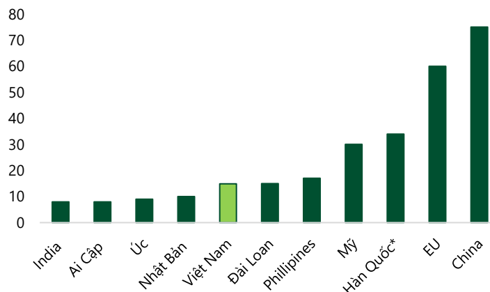
Công suất điện gió mục tiêu đến năm 2030 (GW) của các quốc gia
