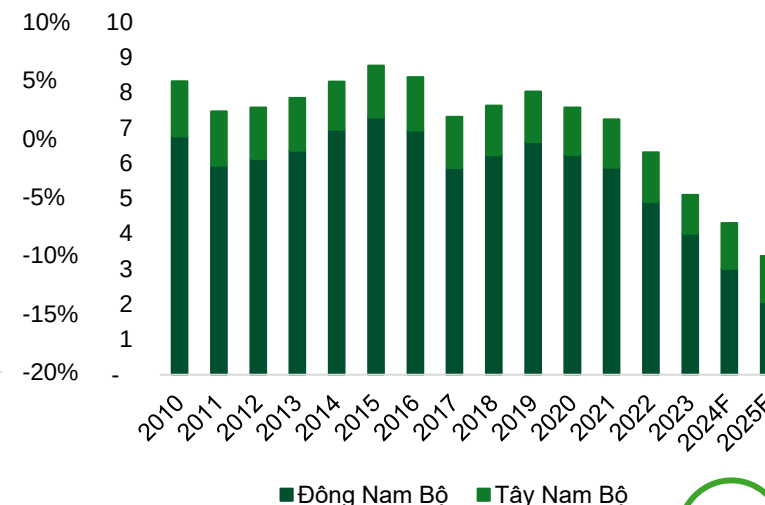
Cơ cấu nguồn khí khai thác trong nước (Tỷ m3)
