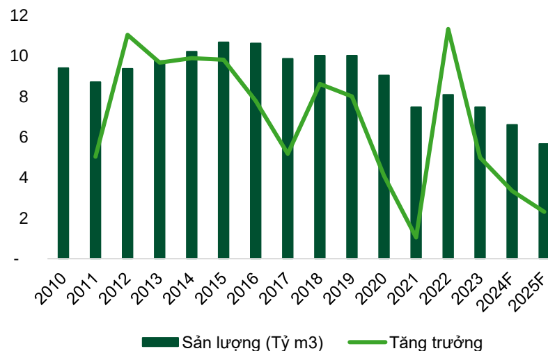
Sản lượng khí khai thác hàng năm ở Việt Nam (Tỷ m3)
