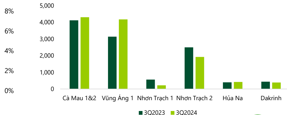
Sản lượng điện của các nhà máy (Triệu kWh)
