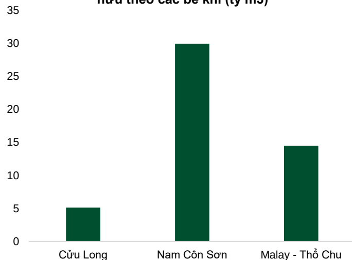
Trữ lượng khí ước tính của các mỏ khí hiện hữu theo các bể khí (tỷ m3)
