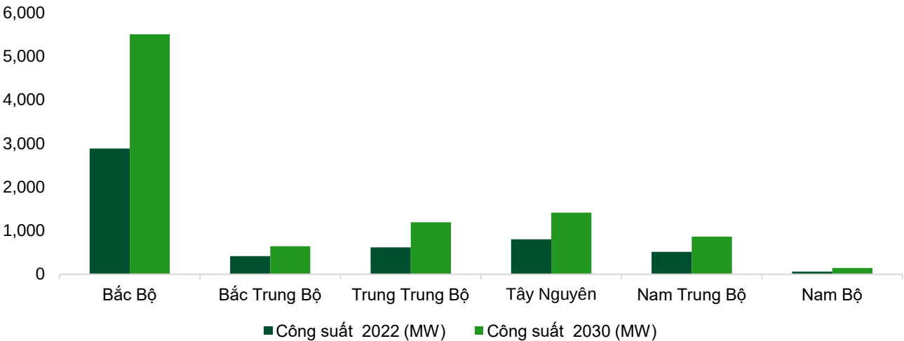
Công suất thủy điện nhỏ (MW)
