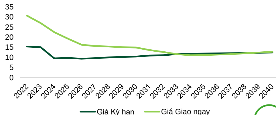
Dự báo giá LNG Asia mua theo Kỳ hạn (Term) và giá Giao ngay (Spot) đến năm 2040 (USD/tr.BTU)
